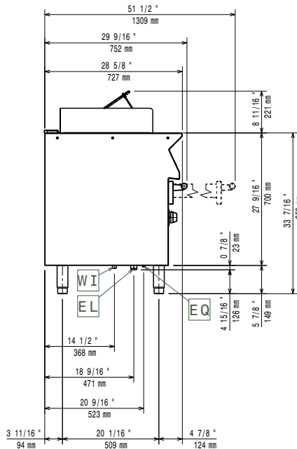
Oldalnézet
